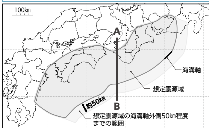
南海トラフ地震臨時想定震源域
