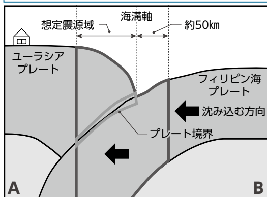
南海トラフ地震臨時想定震源域プレート断面図
