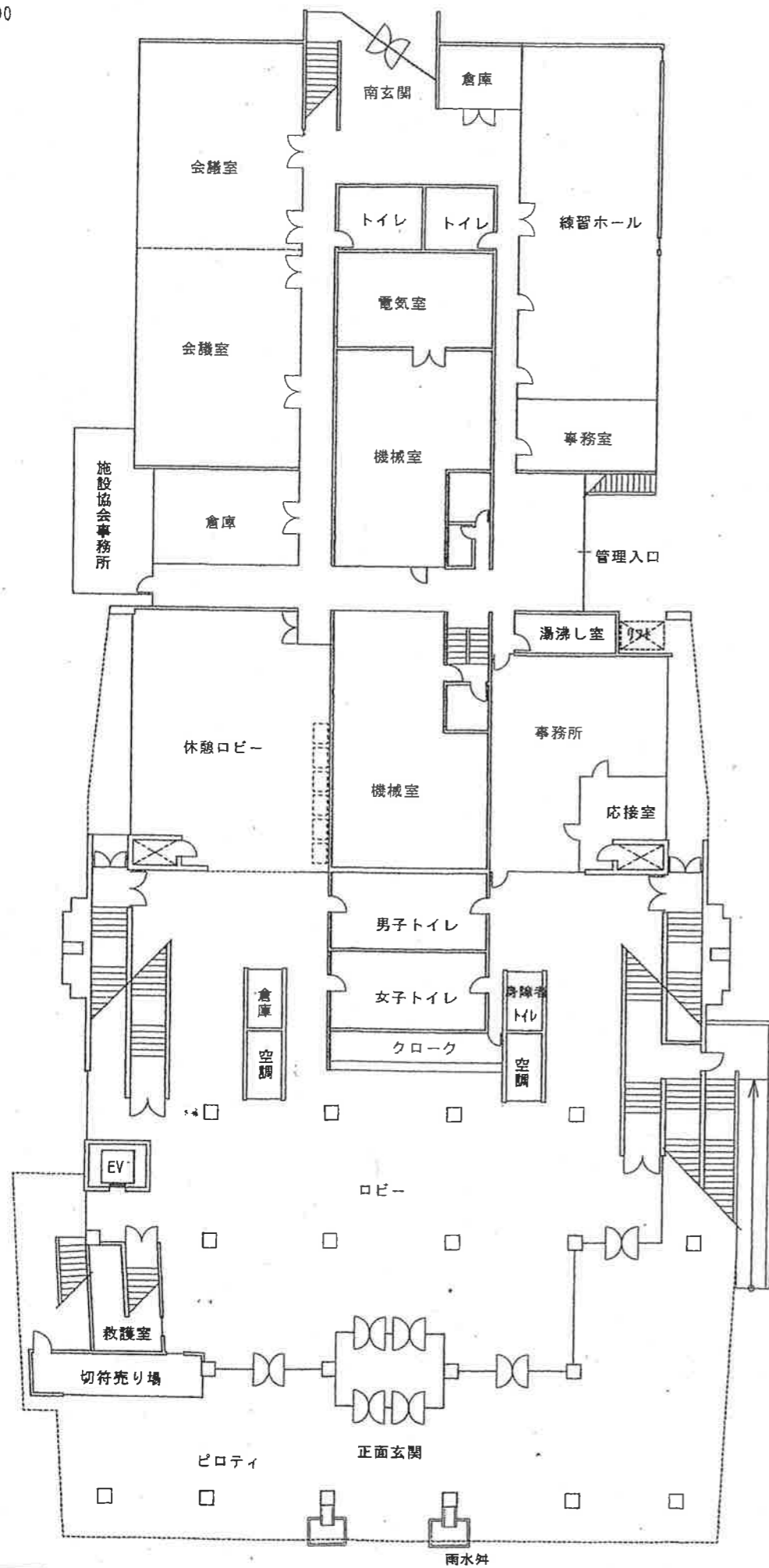
1階平面図
