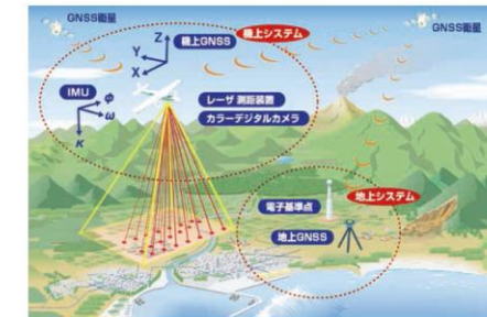
【航空レーザーによる計測イメージ】
