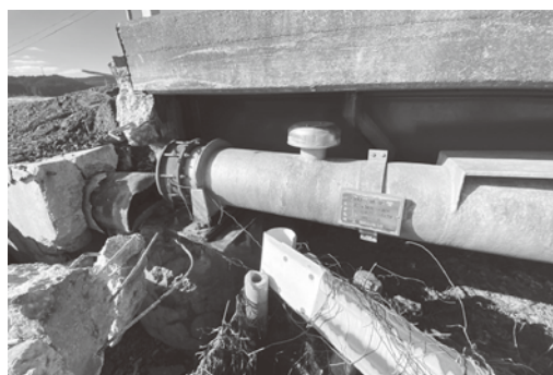
能登半島地震で破損した珠洲市の送水管（日本水道協会提供）。水道施設の被災により、広範囲で断水が発生したと報告されている。
