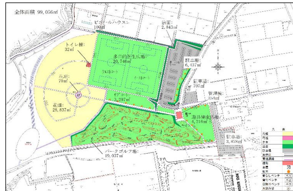
都城市南部ふれあい広場 計画平面図
