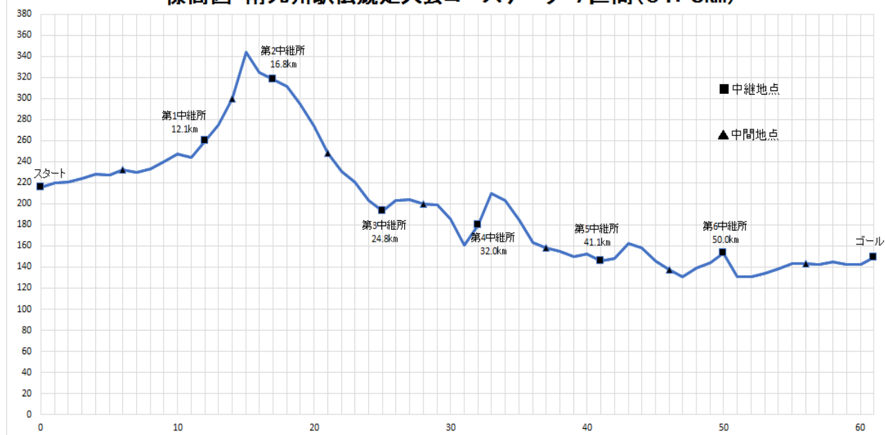
標高図 南九州駅伝競走大会コースデータ 7区間(61.3km)
